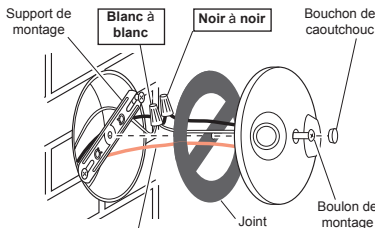
Câblage du projecteur
